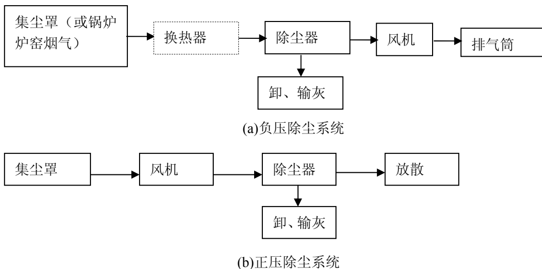
图 1 常见的袋式除尘工艺流程
