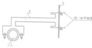
图 3.2.8-3 微差流量测管的安装 1—微差流量测量装置;2—测量管;3—冷箱壁面
